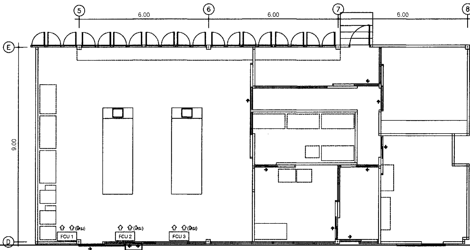
1 แปลนไฟฟ้าระบบเครื่องปรับอากาศ SCALE 1 : 100
