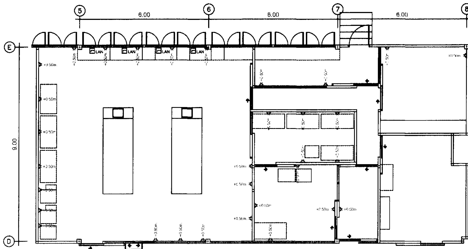
1 แปลนไฟฟ้ากำลัง SCALE 1 : 100
