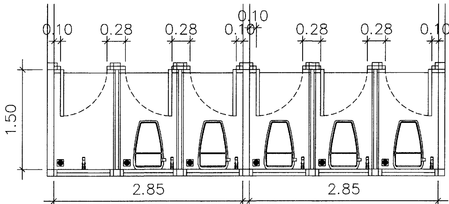
1. แบบขยายห้องน้ำ SCALE 1 : 50
