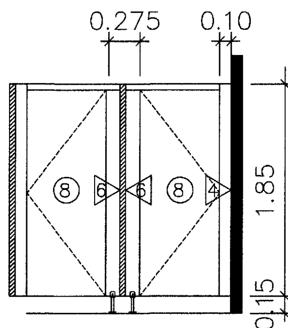
1. รูปตัดห้องน้ำ SCALE 1 : 50
