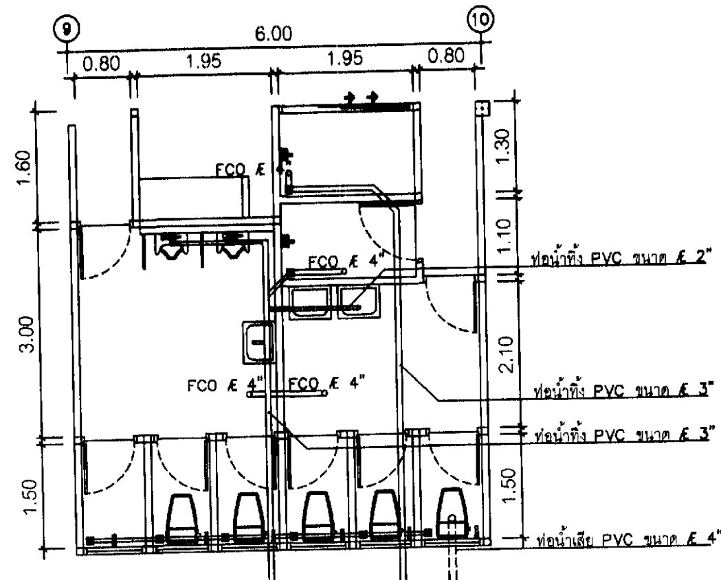
หมายเหตุ : 1. ต่อท่อน้ำทิ้งและท่อน้ำเสียเข้ากับระบบท่อเดิมภายนอกอาคาร 2. ให้ต่อท่ออากาศ (Vent ขนาด 1 1/2") ออกจากนอกอาคาร 1 แปลนระบบท่อน้ำทิ้งและท่อน้ำเสีย SCALE 1 : 75
