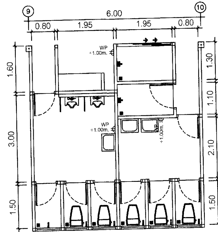
WP. +0.30m. ใต้รับไฟฟ้าคู่ มี GROUND ติดตั้งจากพื้น ตามกำหนดความสูง แบบกันน้ำ
