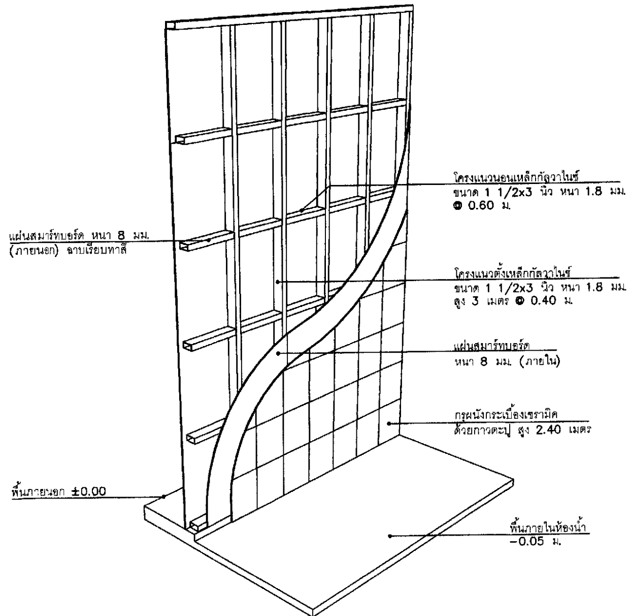
1 แบบขยายการติดตั้งผนังห้องน้ำใหม่ SCALE NTS
