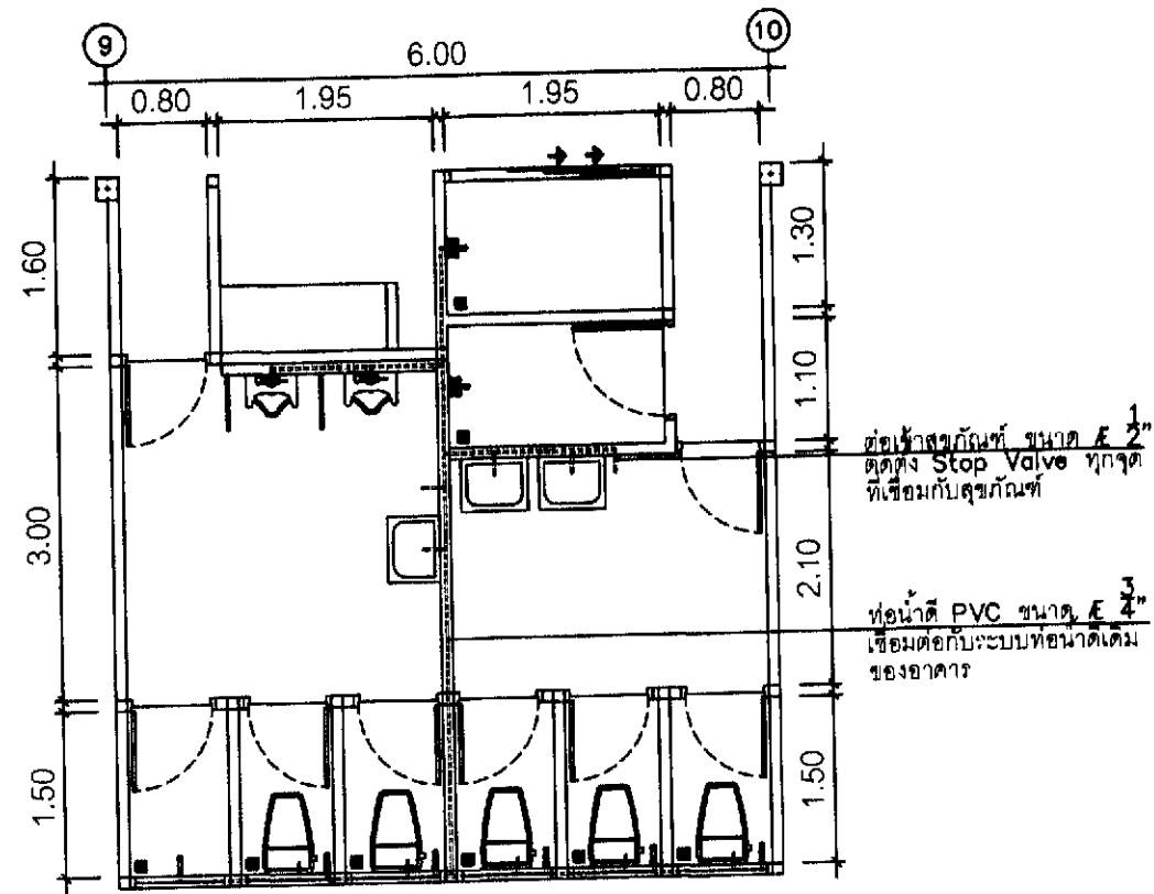
1 แปลนระบบท่อน้ำดี SCALE 1 : 75
