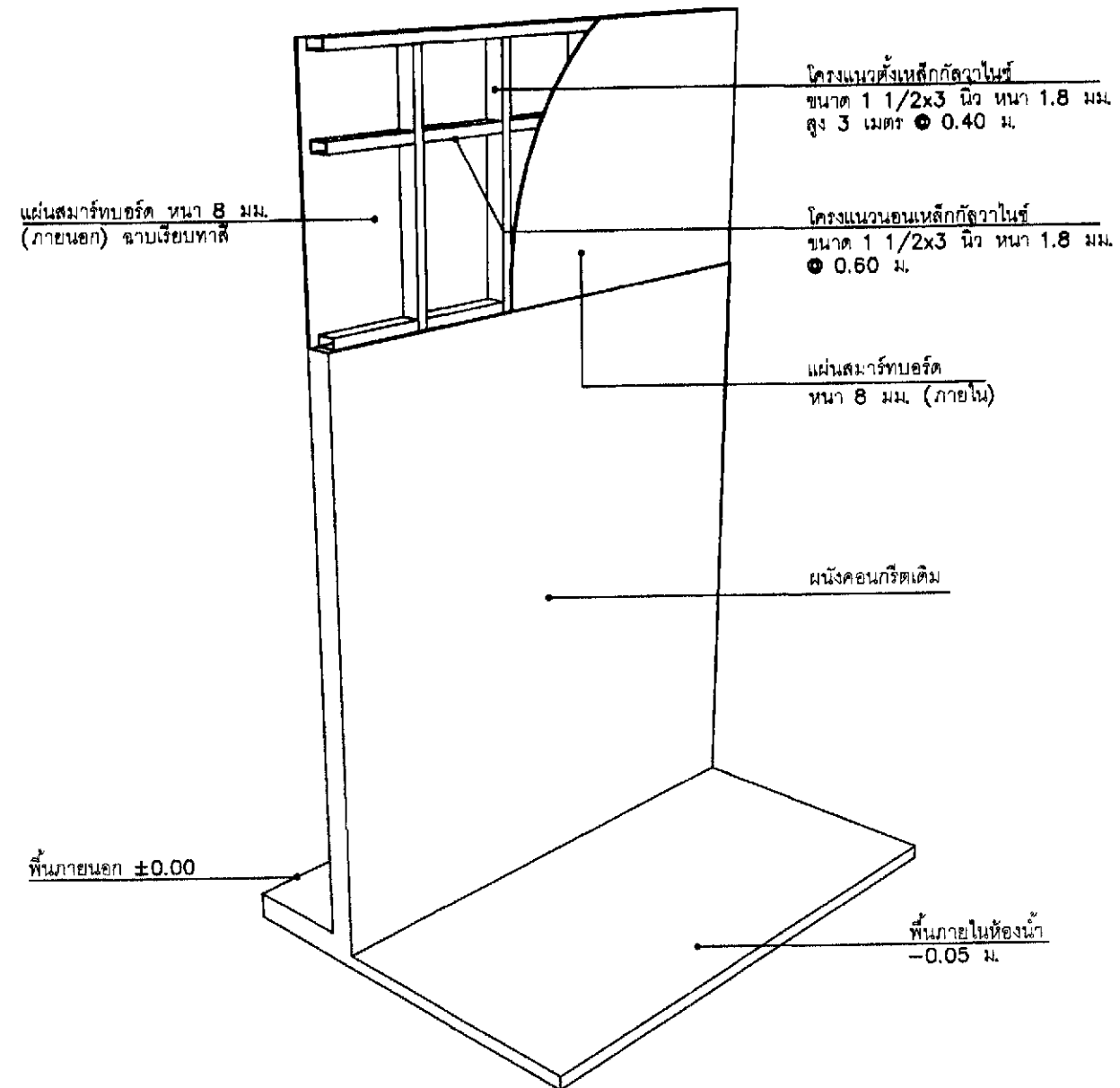
1 แบบขยายการเสริมผนังด้านบนผนังเดิม SCALE NTS
