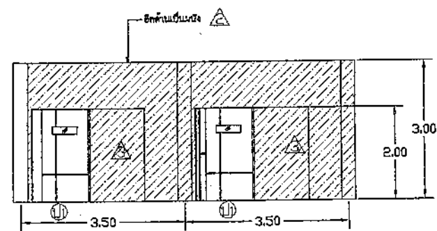
ผนังด้านหน้า
