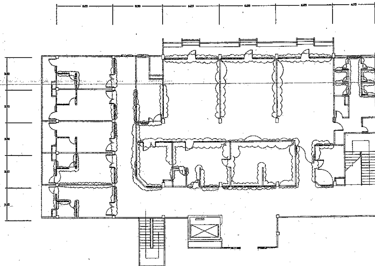
แปลนอาคารครุบาเจ้าเกษมเขมโก ชั้น 4 ก่อนปรับปรุง
