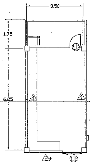
แปลนห้องเก็บของเสีย
