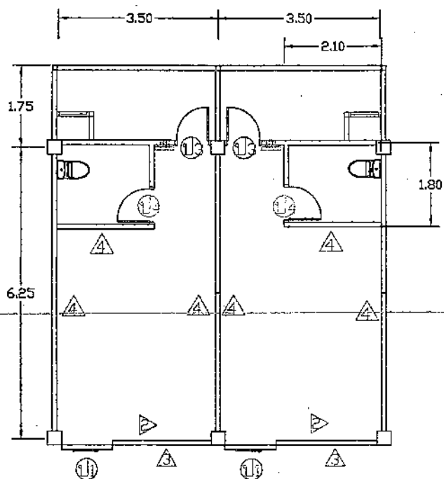
แปลนห้องนอนเวร
