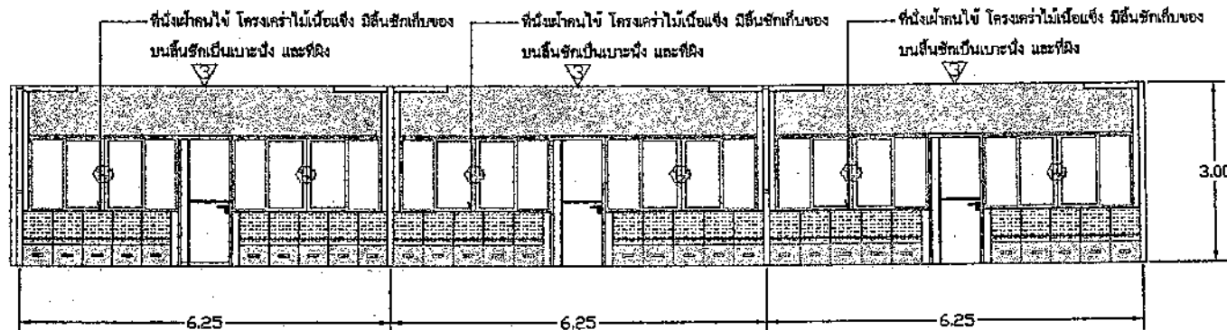
ผนังด้านข้างที่ผู้ป่วยในพิเศษ
