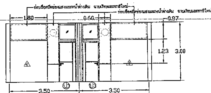
ผนังด้านหลัง
