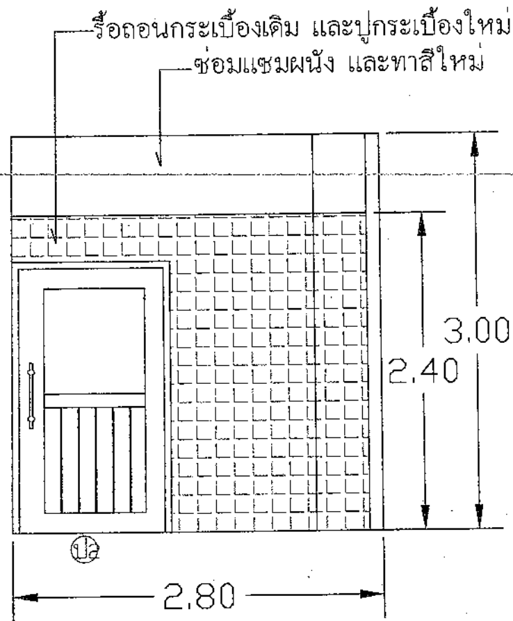
ผนังด้านหน้า
