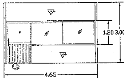
ผนังด้านหน้า Treatment Area
