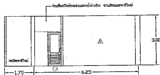
ผนังด้านข้าง
