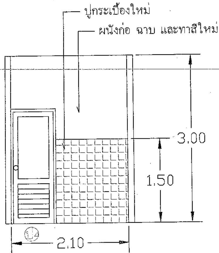
ผนังด้านหน้า
