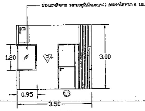
ผนังด้านข้างเคาน์เตอร์พยาบาล
