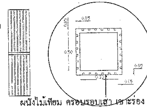
ขยายเสา
