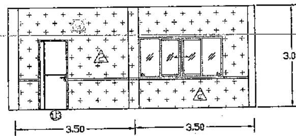
ผนังด้านหลังห้องประชุม
