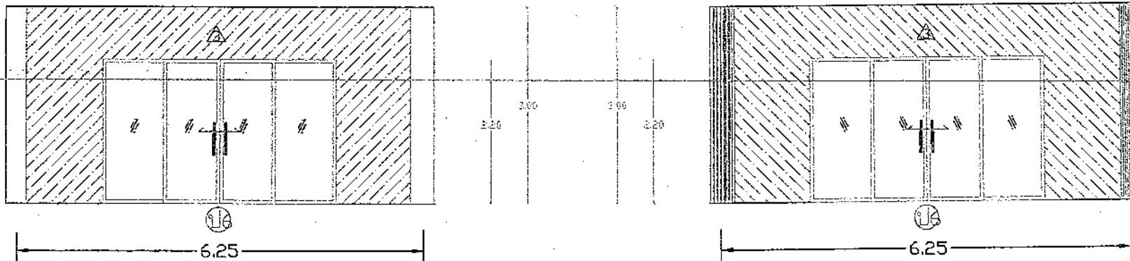
ขยายผนังประตูทางเข้าด้านใน
