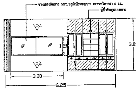
ผนังด้านหลังเคาน์เตอร์พยาบาล
