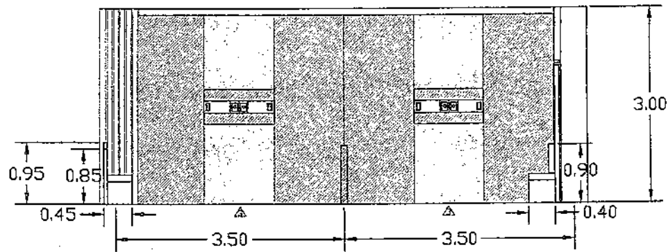
ผนังหัวเตียงที่หักผู้ป่วยในพิเศษ
